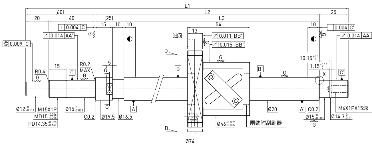
滾珠螺桿資料表
