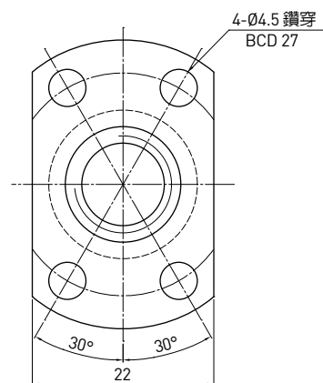
D-D 視圖
