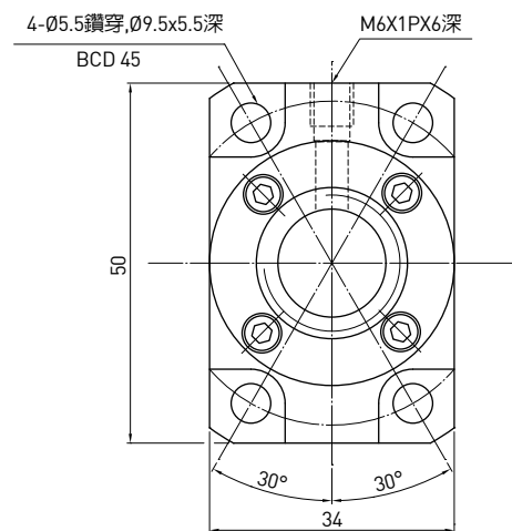
D-D 視圖
