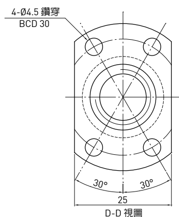
D-D 視圖
