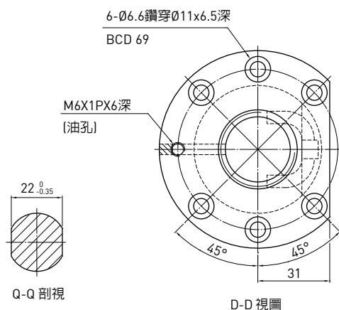
D-D 視圖
