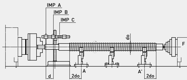
T4: 量測軸承肩部對於螺桿軸AA' 的垂直度 (此量測距離是根據DIN 69051及JIS B1192)
