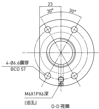
D-D視圖
